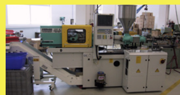
Stroji za brizganje plastike Arburg Allr. 221K, 4 stroji
